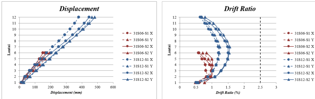
Gambar 5. Displacement dan Drift Arah-X dan Arah-Y Akibat Gempa 2500th Wilayah Surabaya
