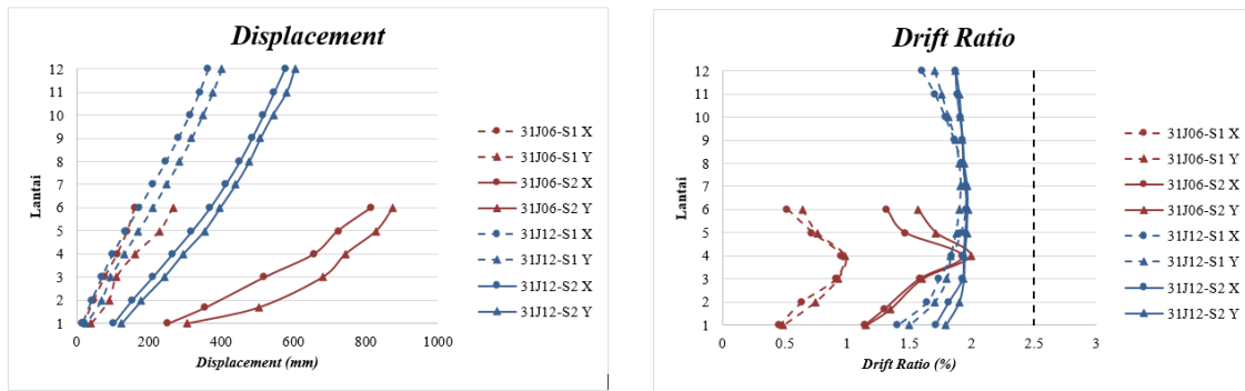
Gambar 5. Displacement dan Drift Arah-X dan Arah-Y Akibat Gempa 2500th Wilayah Jayapura
