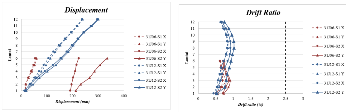
Gambar 2. Displacement dan Drift Arah-X dan Arah-Y Akibat Gempa 100th Wilayah Jayapura
