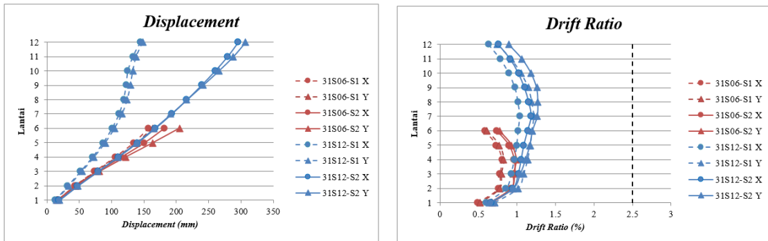
Gambar 3. Displacement dan Drift Arah-X dan Arah-Y Akibat Gempa 500th Wilayah Surabaya
