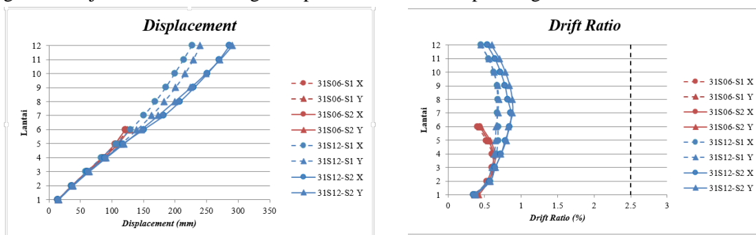
Gambar 1 . Displacement dan Drift Arah-X dan Arah-Y akibat Gempa 100th Wilayah Surabaya
