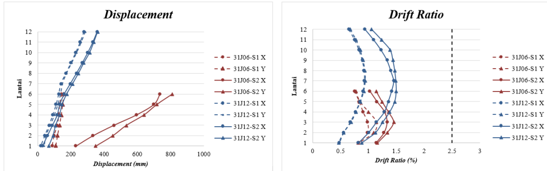
Gambar 4. Displacement dan Drift Arah-X dan Arah-Y Akibat Gempa 500th Wilayah Jayapura
