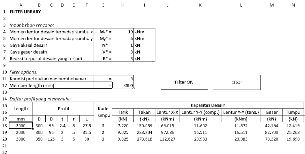
Gambar 9. Tampilan Output Filter dari Library yang Tersimpan
