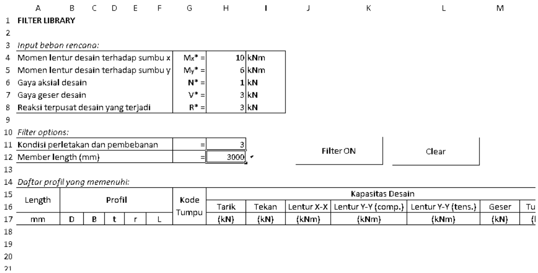
Gambar 8. Tampilan Input Beban Rencana dan Filter Options
