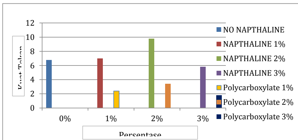
Gambar 2. Hasil kuat tekan mortar dengan superplaztiser umur 7 hari
