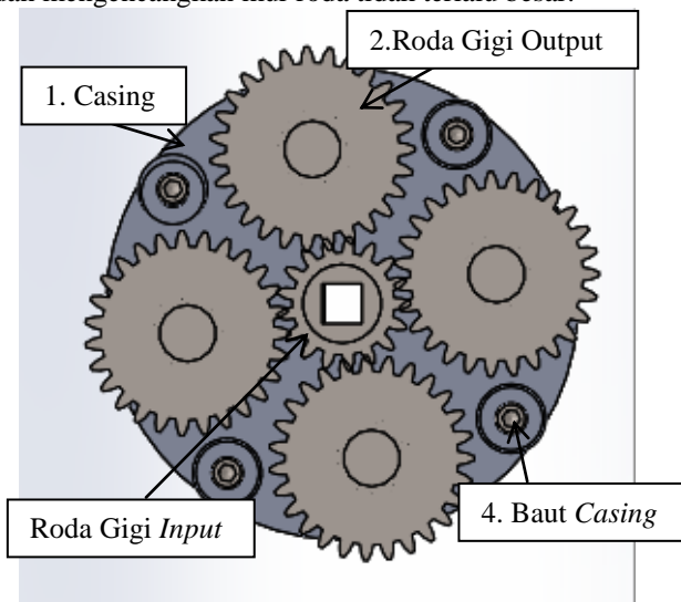
Gambar 3. Desain Alat
