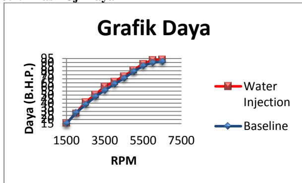
Gambar 6. Grafik Daya Baseline dan Water Injection
