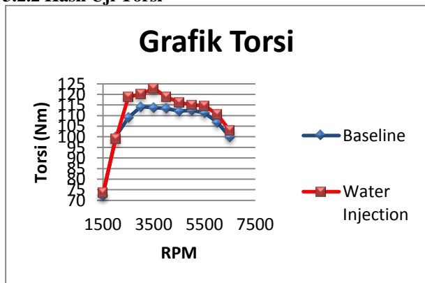
Gambar 7. Grafik Torsi Baseline dan Water Injection
