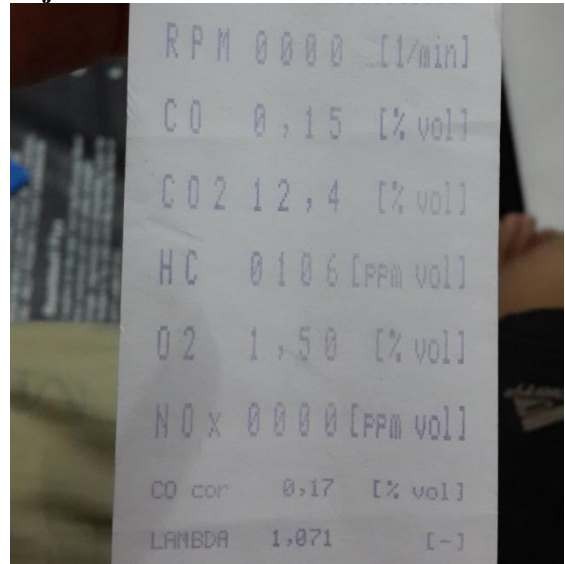
Gambar 8. Hasil Uji Emisi Baseline
