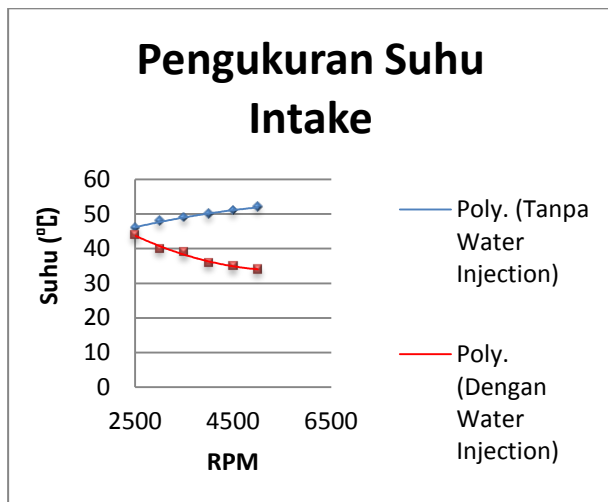
Gambar 10. Grafik Pengukuran Suhu Intake
