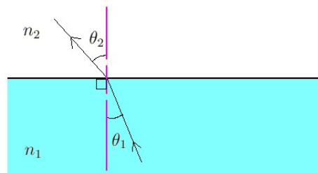
Gambar 1. Ilustrasi pembiasan Snell's law
