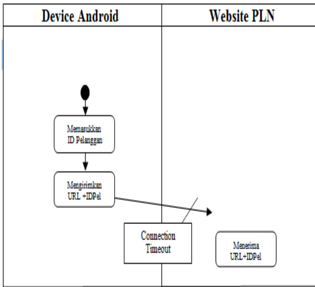
Gambar 3. Timeline protokol komunikasi yang gagal
