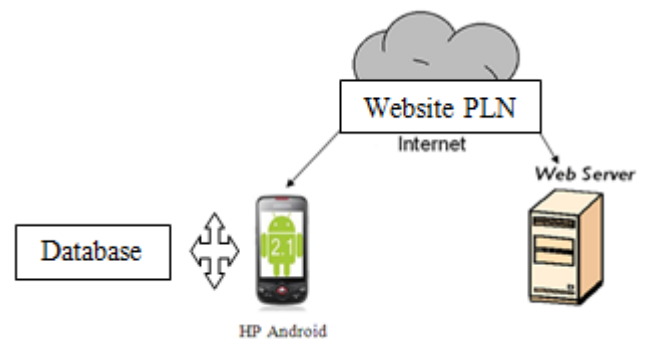
Gambar 1. Arsitektur Aplikasi
