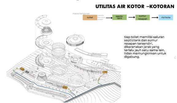
Gambar 5.2. Skema utilitas air kotor dan kotoran
