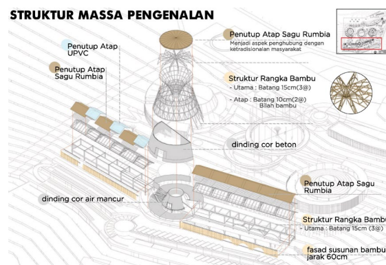
Gambar 4.1. Isometri sistem struktur massa pengenalan
