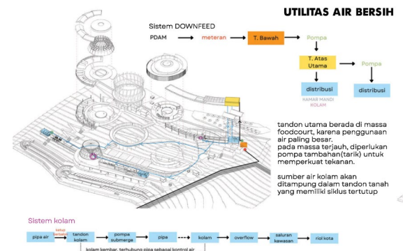
Gambar 5.1. Isometri utilitas air bersih
