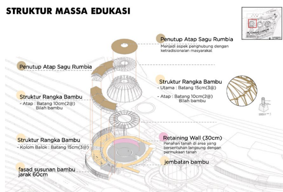
Gambar 4.3. Isometri sistem struktur massa edukasi
