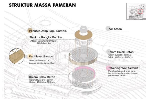
Gambar 4.2. Isometri sistem struktur massa Pameran
