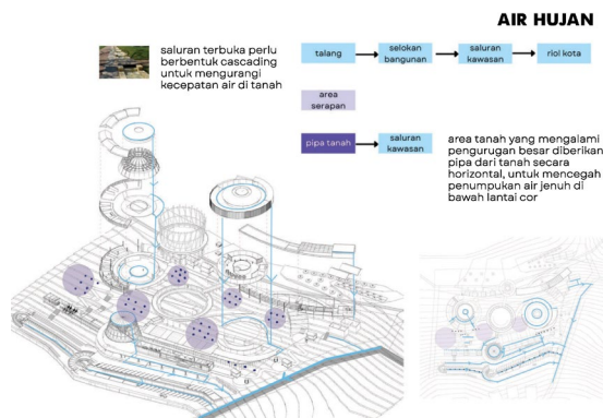
Gambar 5.3. Skema utilitas air hujan
