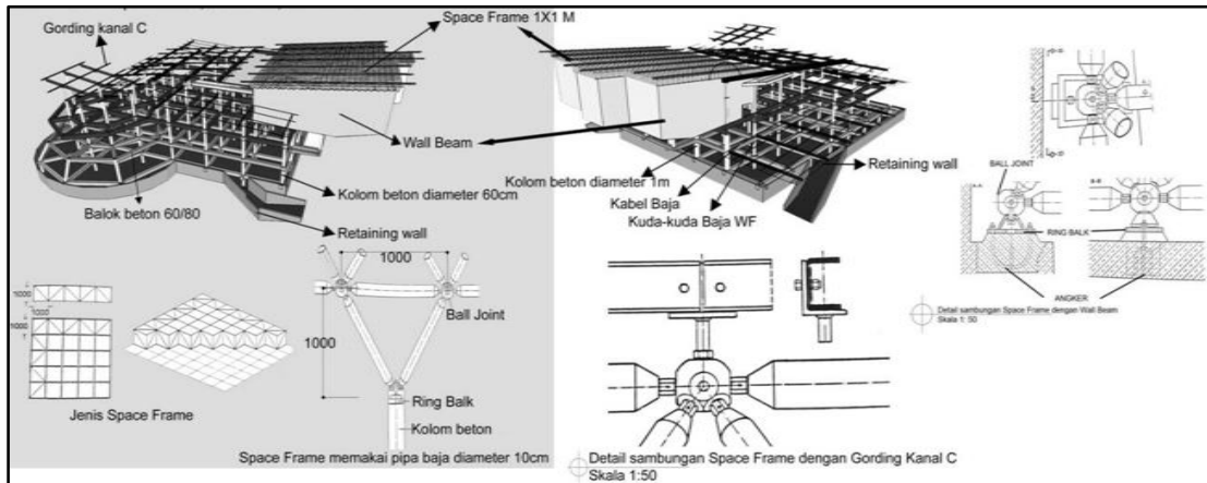
Gambar 15. Detail Space Frame pada atap bangunan
