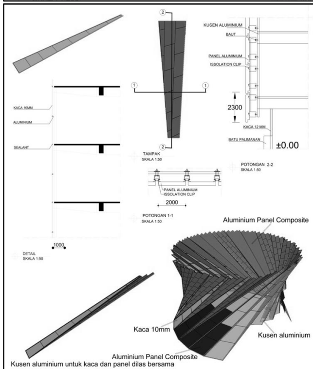
Gambar 16: Atas: Potongan bangunan feminim Samping: Detail fasade pada bangunan feminim
