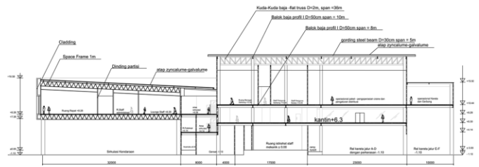
Potongan B-B Skala 1:200 Gambar 2.7 Potongan bangunan.
