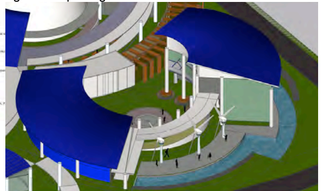
Gambar 2.17. Galeri Energi
