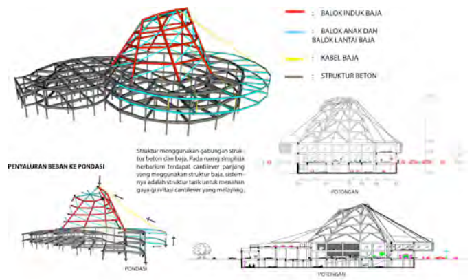
Gambar 2.13 Sistem Struktur Bangunan
