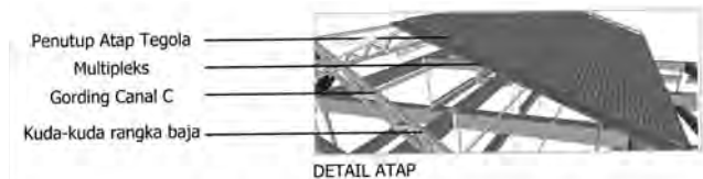
Gambar. 2.25 Detail Penutup Atap
