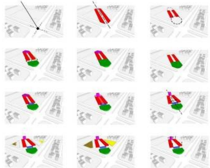
Gambar 2.4 Transformasi Massa
