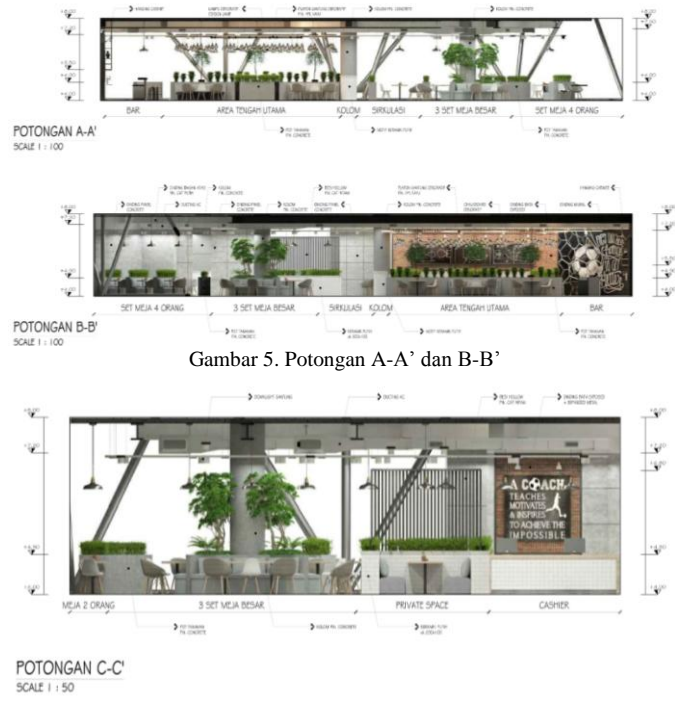
Gambar 6. Potongan C-C'
