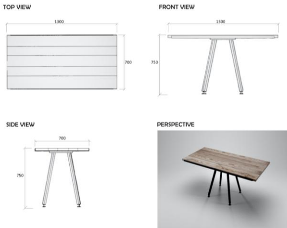
Gambar. 27. Detail Perabot Meja Makan
