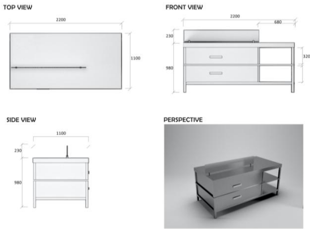
Gambar. 26. Detail Perabot Meja Dapur
