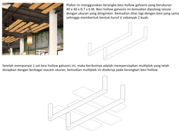
Gambar. 32. Detail Plafon
