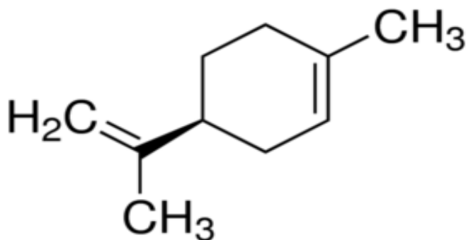
Gambar. 2. Rangkaian senyawa kimia dari limonene
