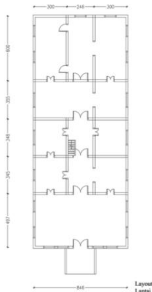
Gambar 14. Layout Malige , Suku Wolio
