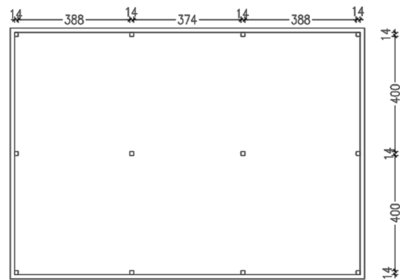
Gambar 18. Layout Rumah adat Suku Wolio.
