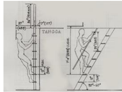
Gambar 6. Dimensi Tangga Sumber : Ching (1996, p. 228)
