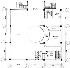
Gambar 11. Tapak Dalam Bangunan Lantai 3
