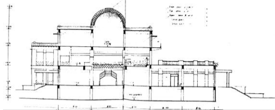
Gambar 12. Tampak Potongan Bangunan
