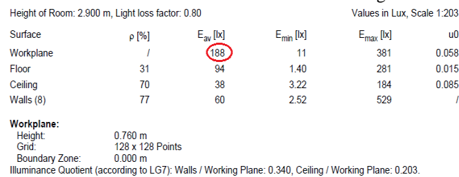
Gambar 3. Daftar hasil perhitungan luminasi pada kantor Sequislife di lantai 8 [2].
