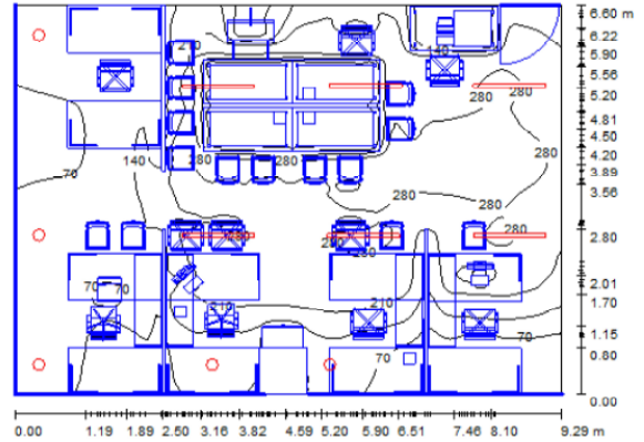
Gambar 14. Model replika lay out penyebaran cahaya pada kantor Sequislife di lantai 1 [2].
