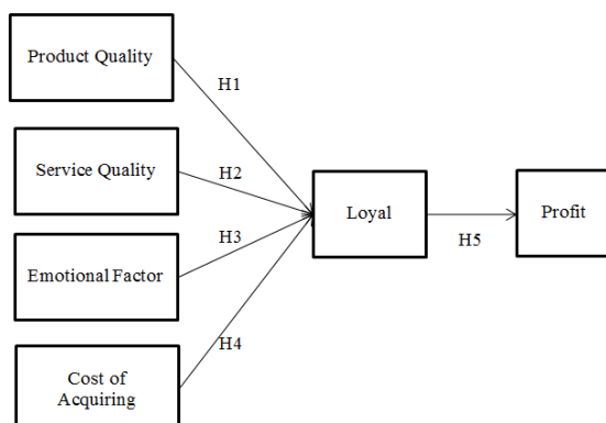
Gambar 1 Kerangka Berpikir
